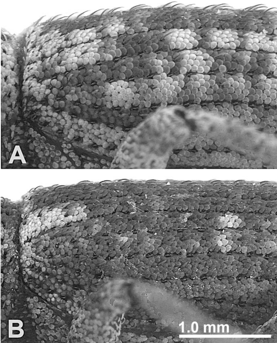
Fig. 3. A: Simo variegatus (Boheman, 1843): Switzerland, Valais: Chelin. — B: Simo hirticornis (Herbst, 1795): Italy, Piemonte: Gran Paradiso.
